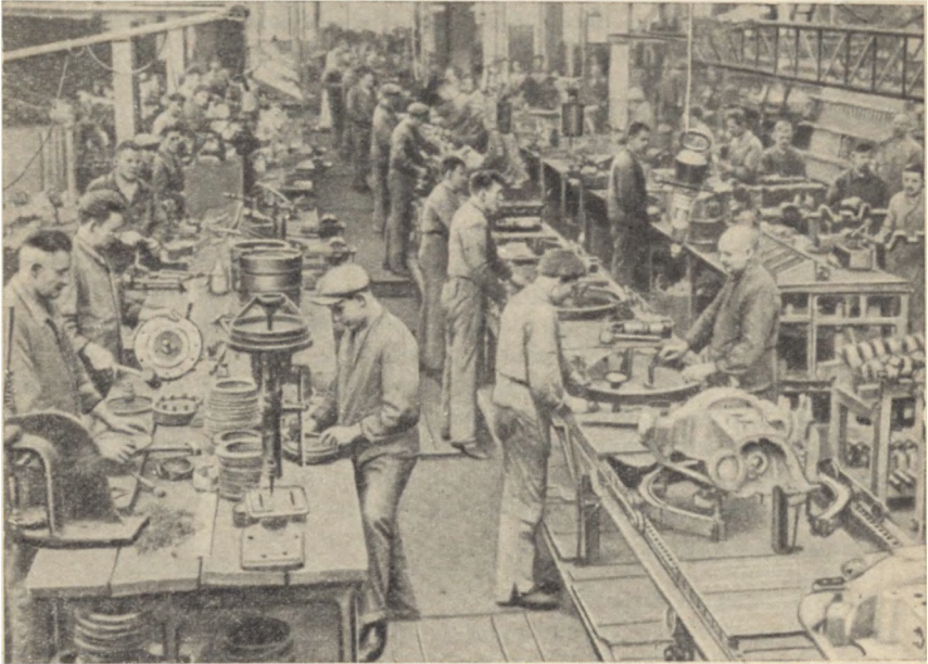
Сборка шестицилиндровых моторов на конвейере завода Опеля в Руссельсгейме, 1928 г
